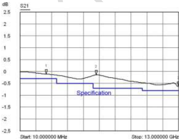
141-01-01-100R 的典型 S21 指标:
