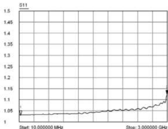
14-03-07-1000LIM 的典型 S11 指标:
