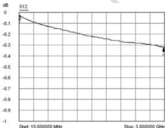
14-03-07-1000LIM 的典型 S21 指标:
